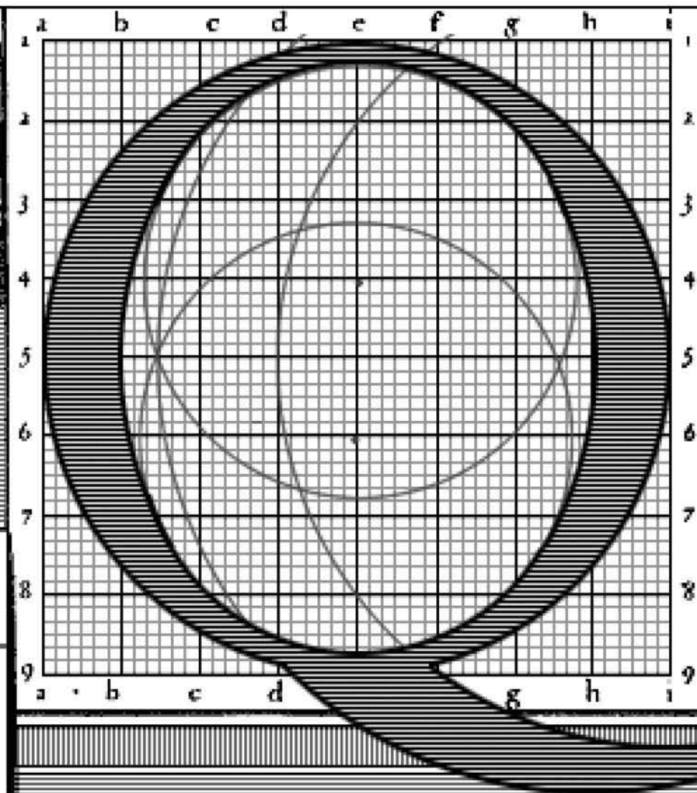
Construction de la lettre Q
